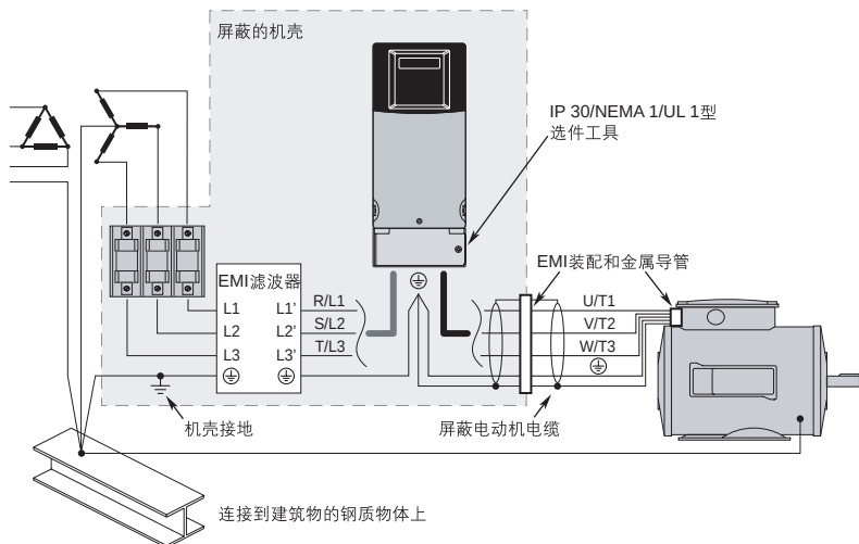
图 1.8 连线和接地
