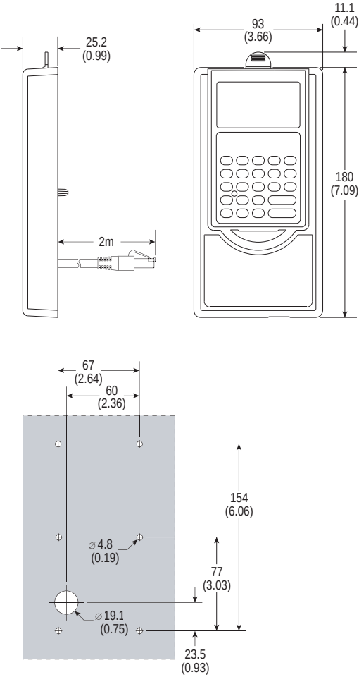
图 B.9 NEMA 1 型前盖工具- 尺寸以毫米和(英寸) 为单位。 目录号: 22-HIM-B1
