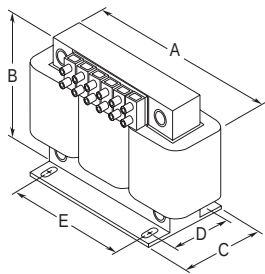
图 B.5 Bulletin 1321-3R系列线路电抗器 尺寸以毫米和(英寸)为单位。重量以千克和(磅)为单位。
