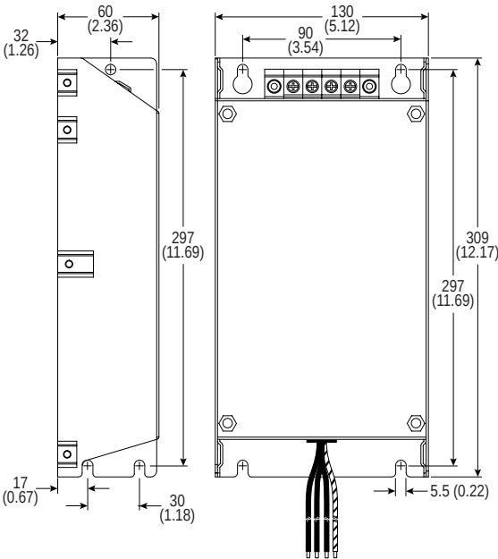
图 B.7 EMC线路滤波器-尺寸以毫米和(英寸)为单位。
