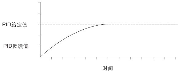
图D.3 振荡—欠阻尼
