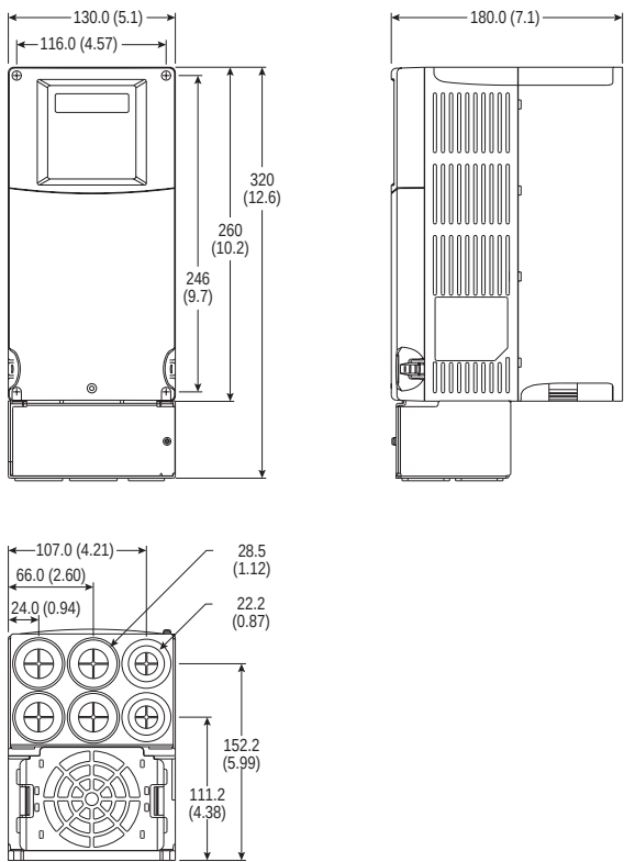
图 B.1 PowerFlex 400 C 型框架变频器 尺寸以毫米和 (英寸) 为单位。
