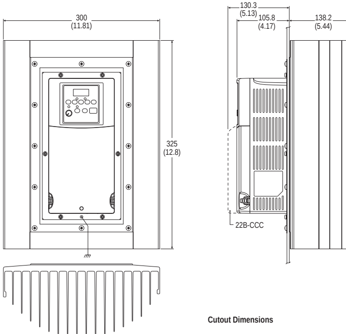
图 B.4 PowerFlex 400C 型框架法兰式安装变频器 尺寸以毫米和(英寸)为单位。
