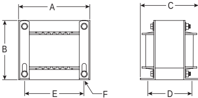
图B.6 Bulletin 1321-直流母线电抗器尺寸以毫米和(英寸)为单位。重量以千克和(磅)为单位。
