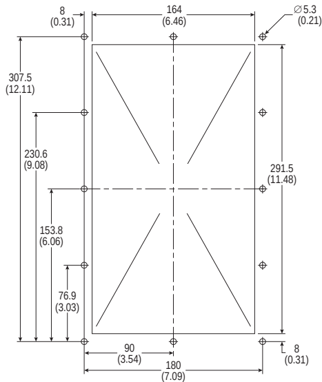
Cutout Dimensions
