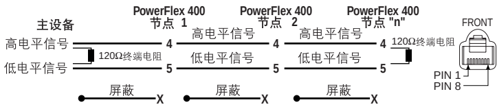
图 E.1 网络布线图
