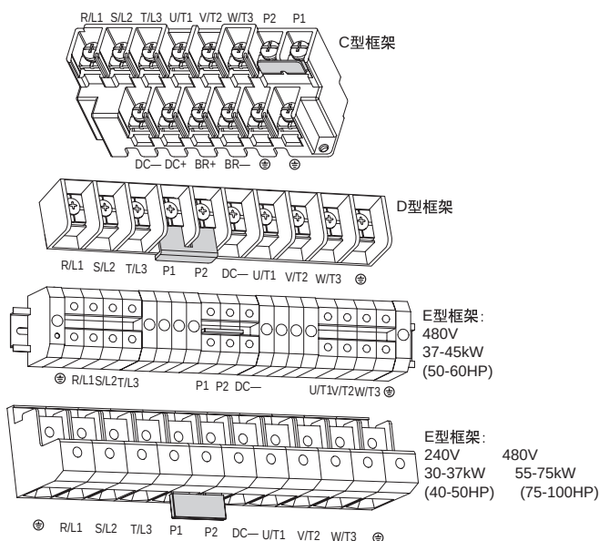
图 1.6 电源端子块
