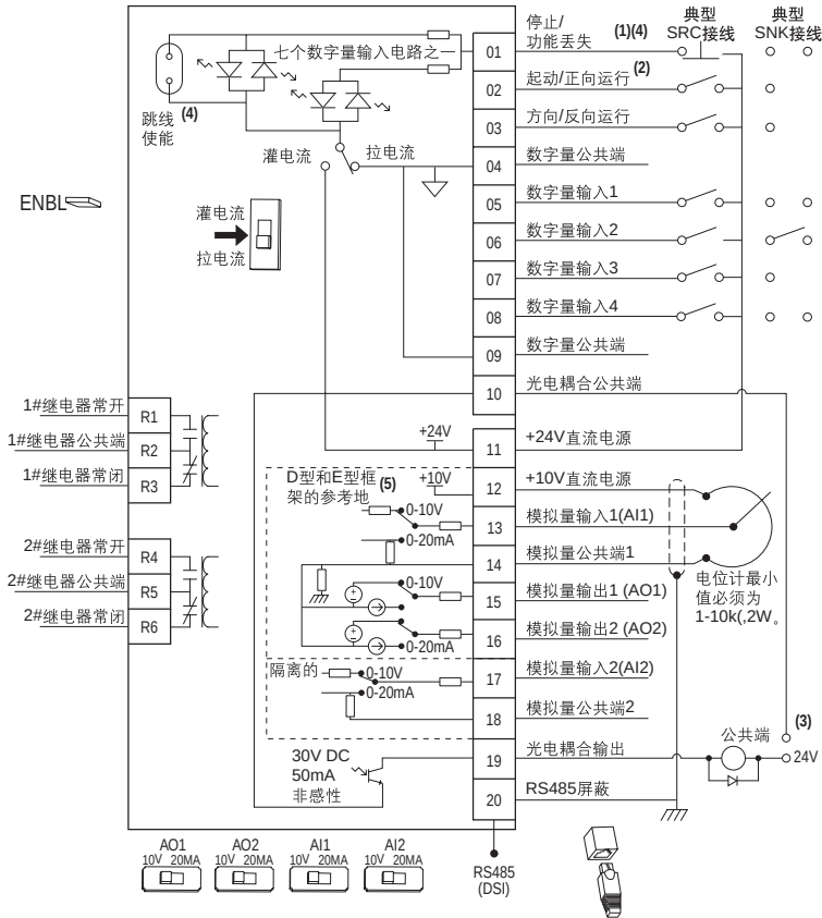
图1.7 控制接线功能图
