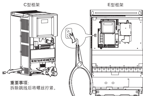
图1.4 跳线位置
