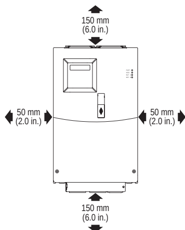
图1.2 D型框架和E型框架安装间距
