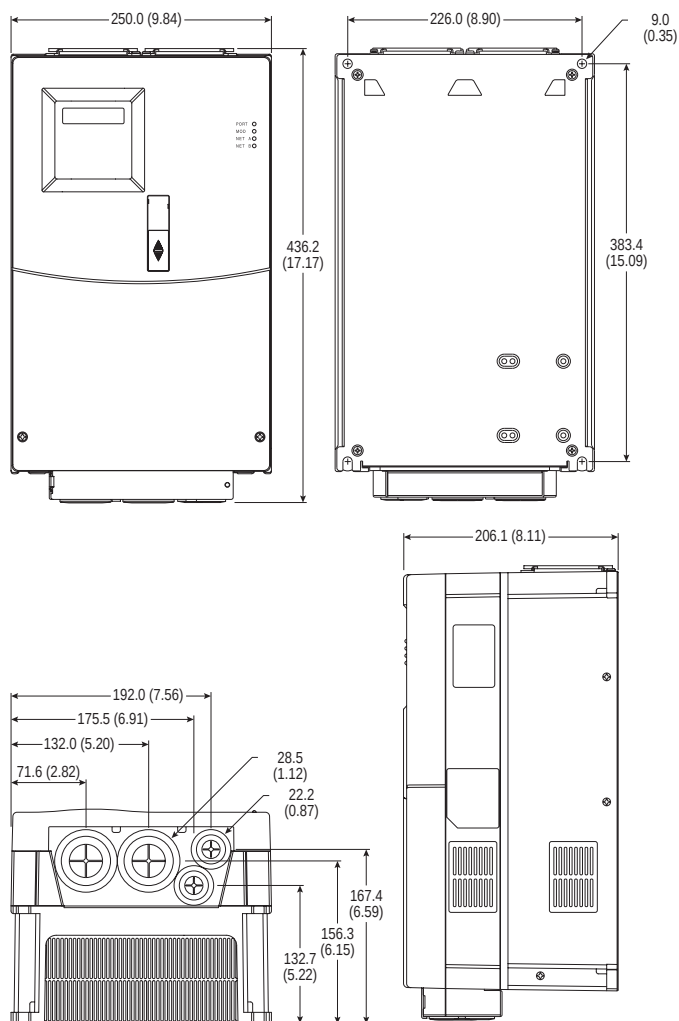
图 B.2 PowerFlex 400 D型框架变频器-尺寸以毫米和(英寸)为单位。
