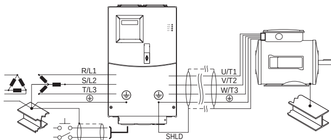
图 1.5 典型接地
